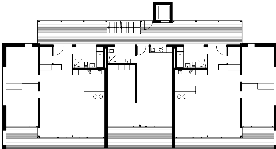
Grundriss Erdgeschoss
